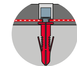
Innensechskantschraube + Dübel
