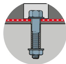
Maschinenschraube + Mutter
