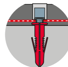
Innensechskantschraube + Dübel
